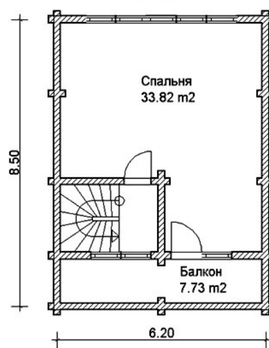
ПЛАН МАНСАРДЫ
