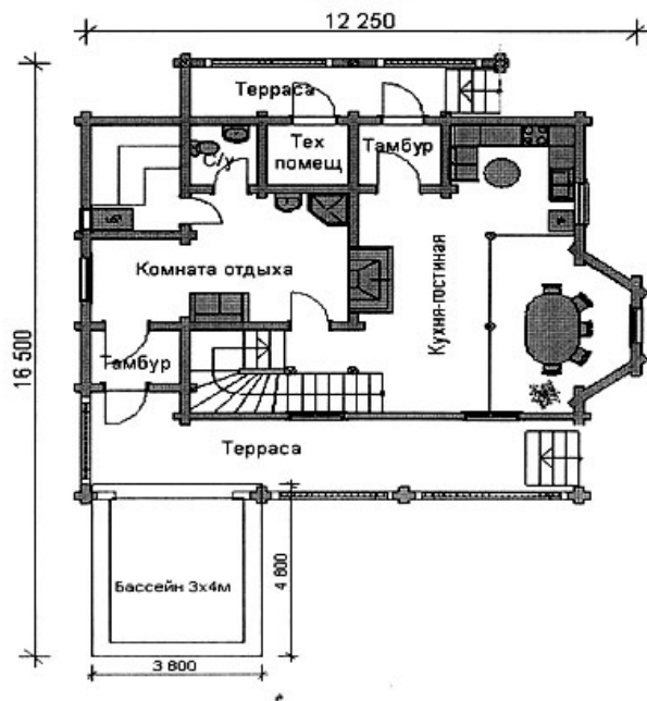
План 1 этажа
