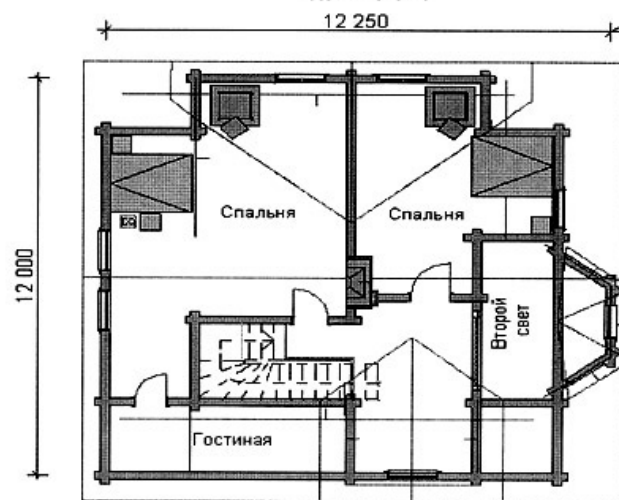
План 2 этажа
