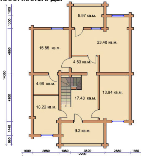
ПЛАН МАНСАРДЫ
