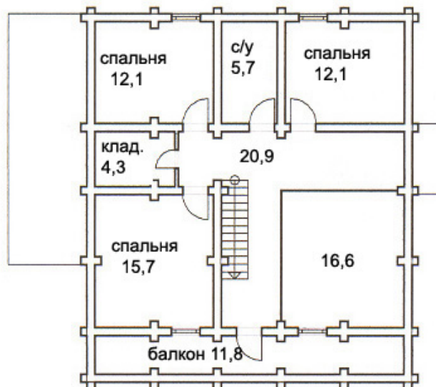
План мансарды
