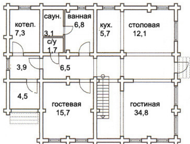
План 1 этажа
