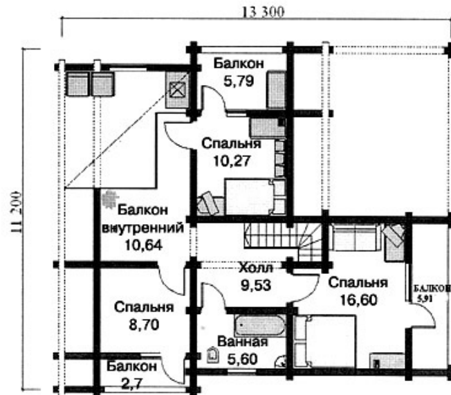
План 2 этажа
