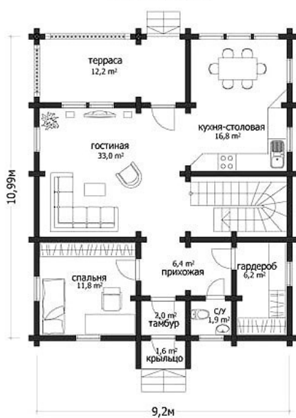
ПЛАН 1-ГО ЭТАЖА
