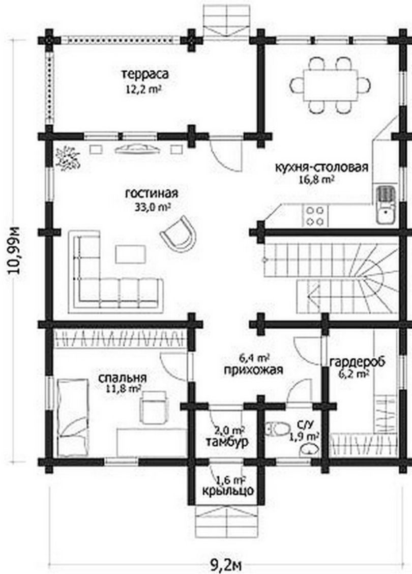
ПЛАН 1-ГО ЭТАЖА
