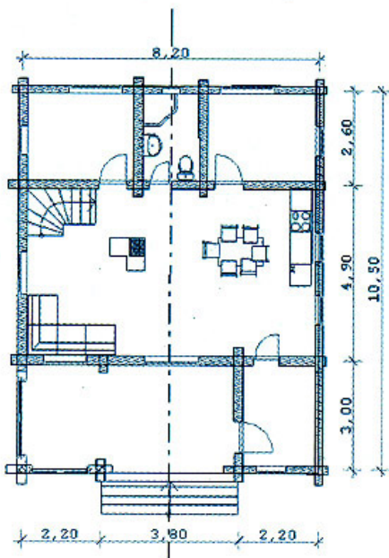
План 1 этажа
