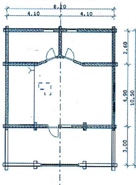
План 2 этажа
