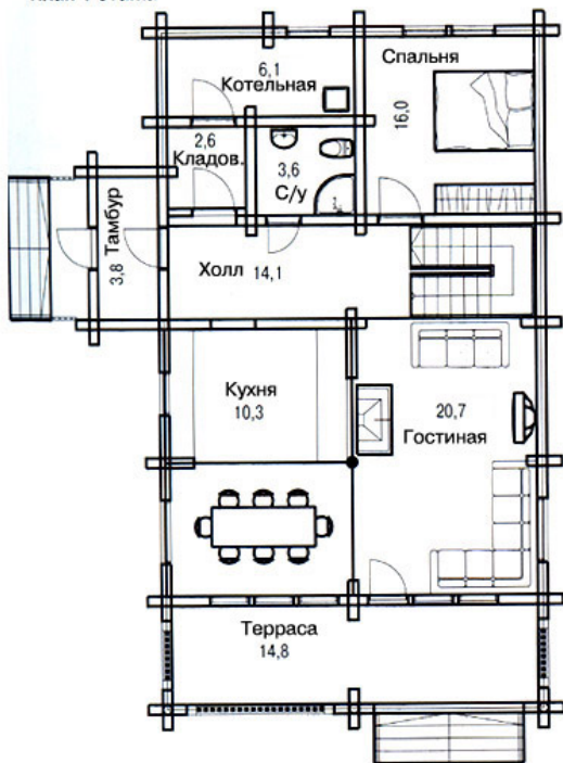
План 1 этажа
